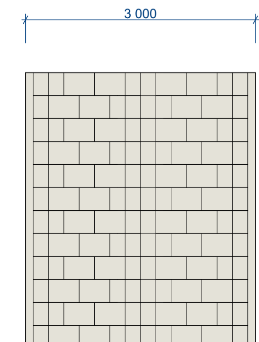
SCHÉMA KLADENIA DLAŽBY SP1
